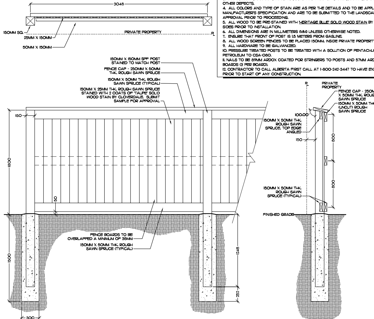
1 L1 1.8M WOOD SCREEN FENCE SCALE: N.T.S.
